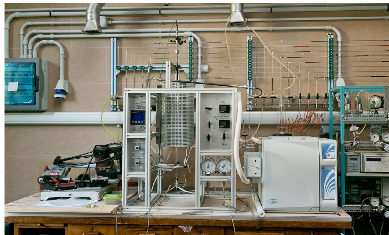
▲ Проточная каталитическая установка конверсии \text{CO}_2 (оснащение комнаты произведено на средства гранта РФФ)
